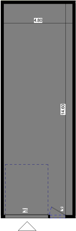
PLAN RDC
